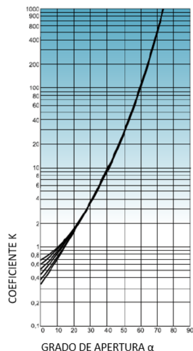
DIAGRAMA DE PÉRDIDA DE CARGA EN FUNCIÓN DEL GRADO DE APERTURA
