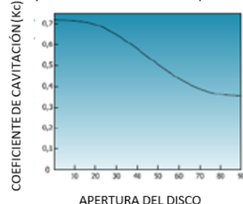
VALORES DE CAVITACIÓN (αc) (Coeficiente de cavitación)
